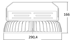
ALUMAX/N-XL-200W
