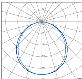
N/OPALPC-IP65-55W
