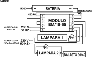
Fig. 4: SISTEMA PERMANENTE CON 2 LAMPARAS EN SERIE
