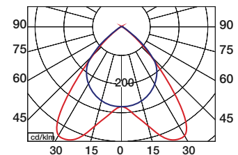
NX-T5 4x14W
