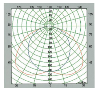
ALUX 2x54 W.
