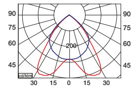
NT-5 4x14 W.
