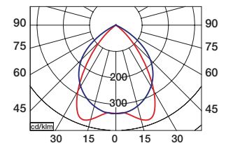
T5/MR 4x14 W.
