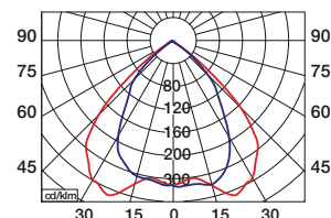
LUXUS 269/A - 2x26W
