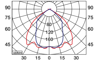
LUXUS 243/BR - 2x26W
