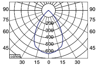
DLUX-IP44-G12 1x150W HIT-CE
